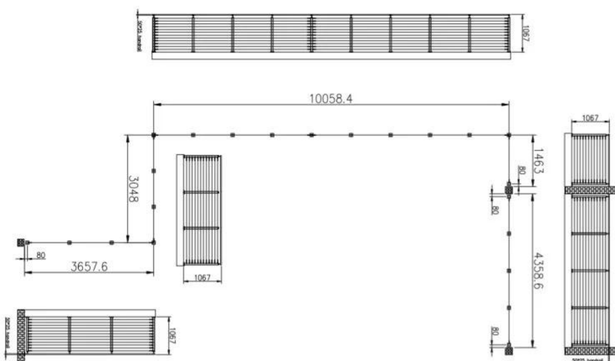
Rysunek balustrady kablowej i słupka poręczy
