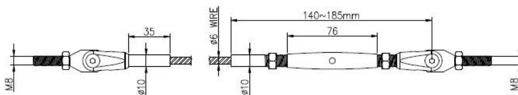
2) Cable tensioner T804 dimension
