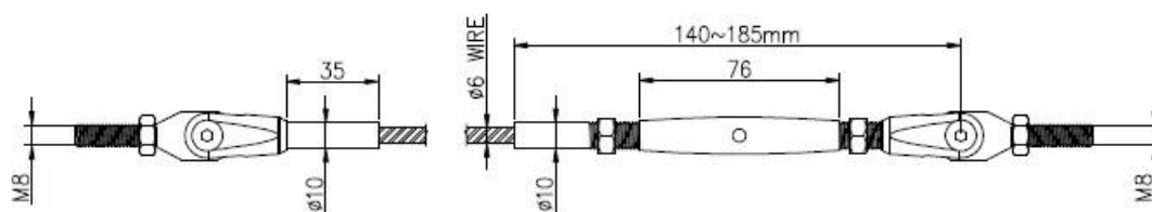
Esticador de cabo T803 tamanho
