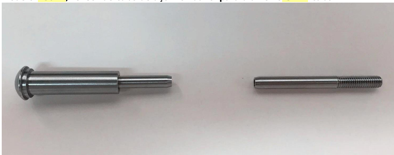
Modelo T807A, tensor de cabo de aço inoxidável para diâmetro 3mm cabo:
