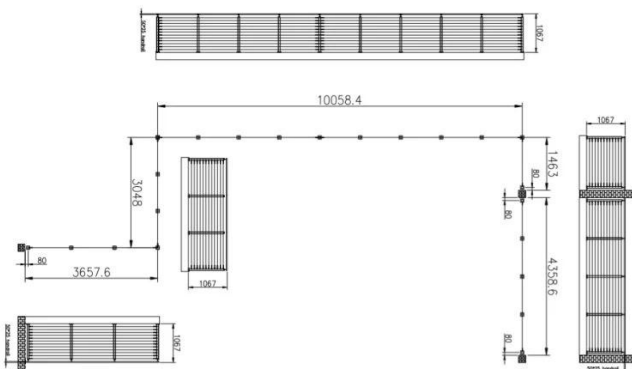
Desenho de guarda-corpo e poste de guarda-corpo
