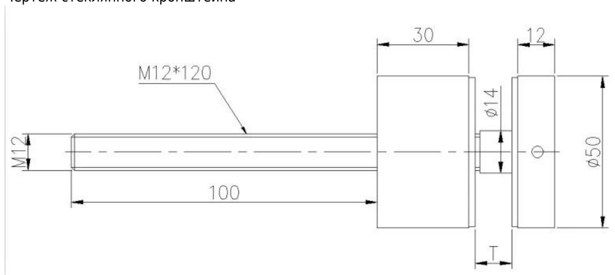
Чертеж стеклянного кронштейна-
