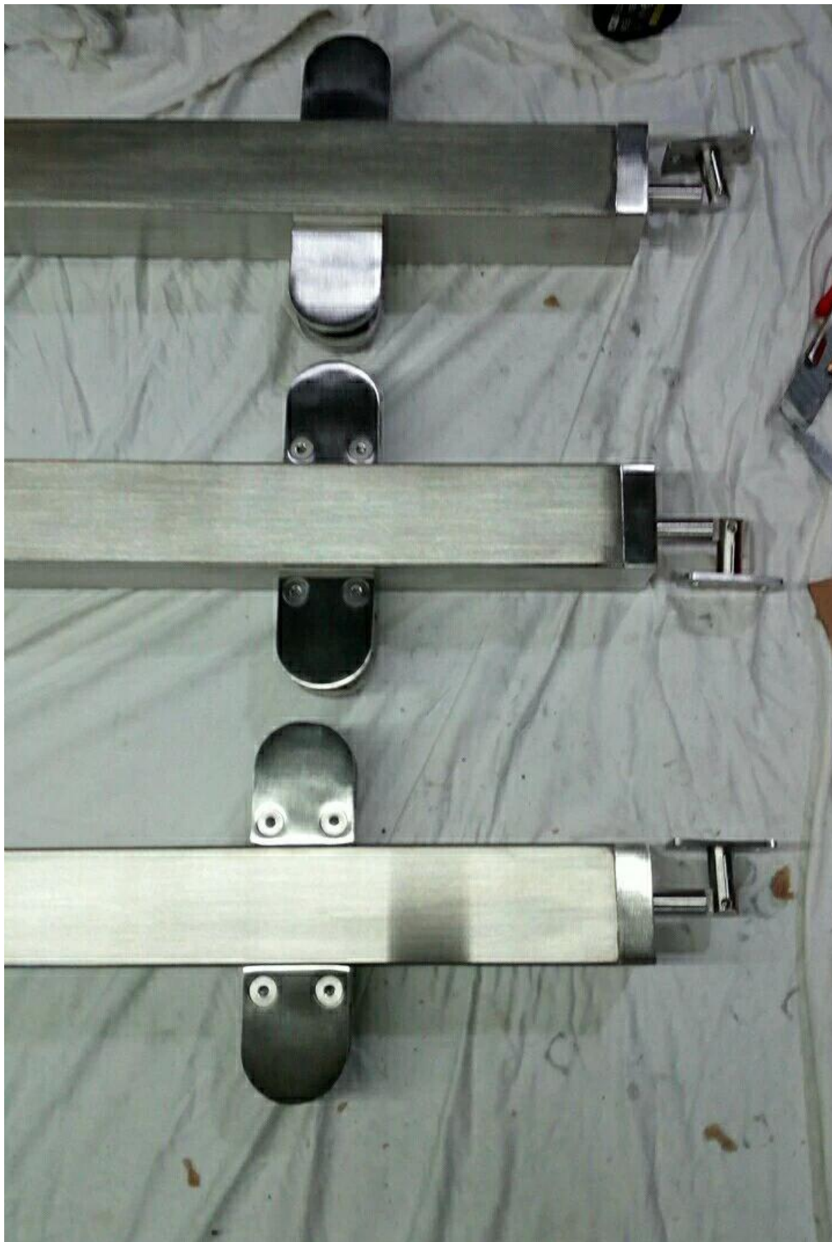
Крепление фасции / боковое поручение поручней перила Сначала соедините пластину сбоку, затем прикрепите ее двумя винтами
