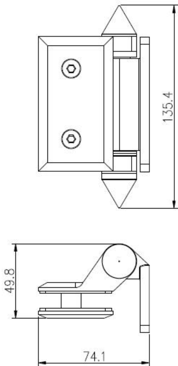
Стекло G-R на петлю с круглой стойкой
