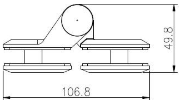
G-W стекло к квадратной стойке / настенной петле
