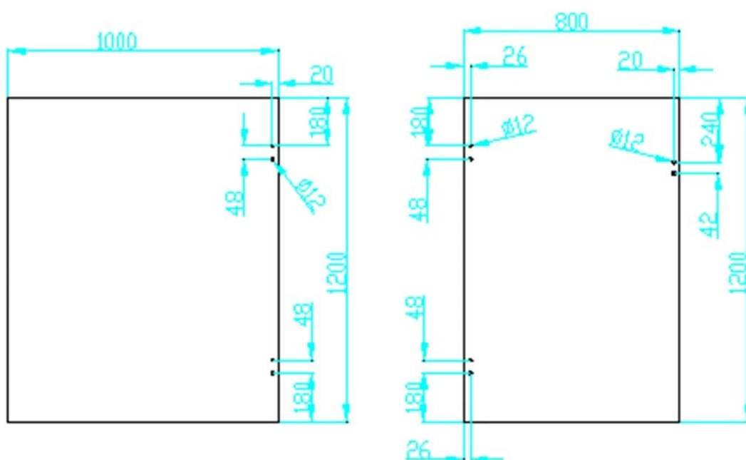
Чертеж для размера отверстия для стекла
