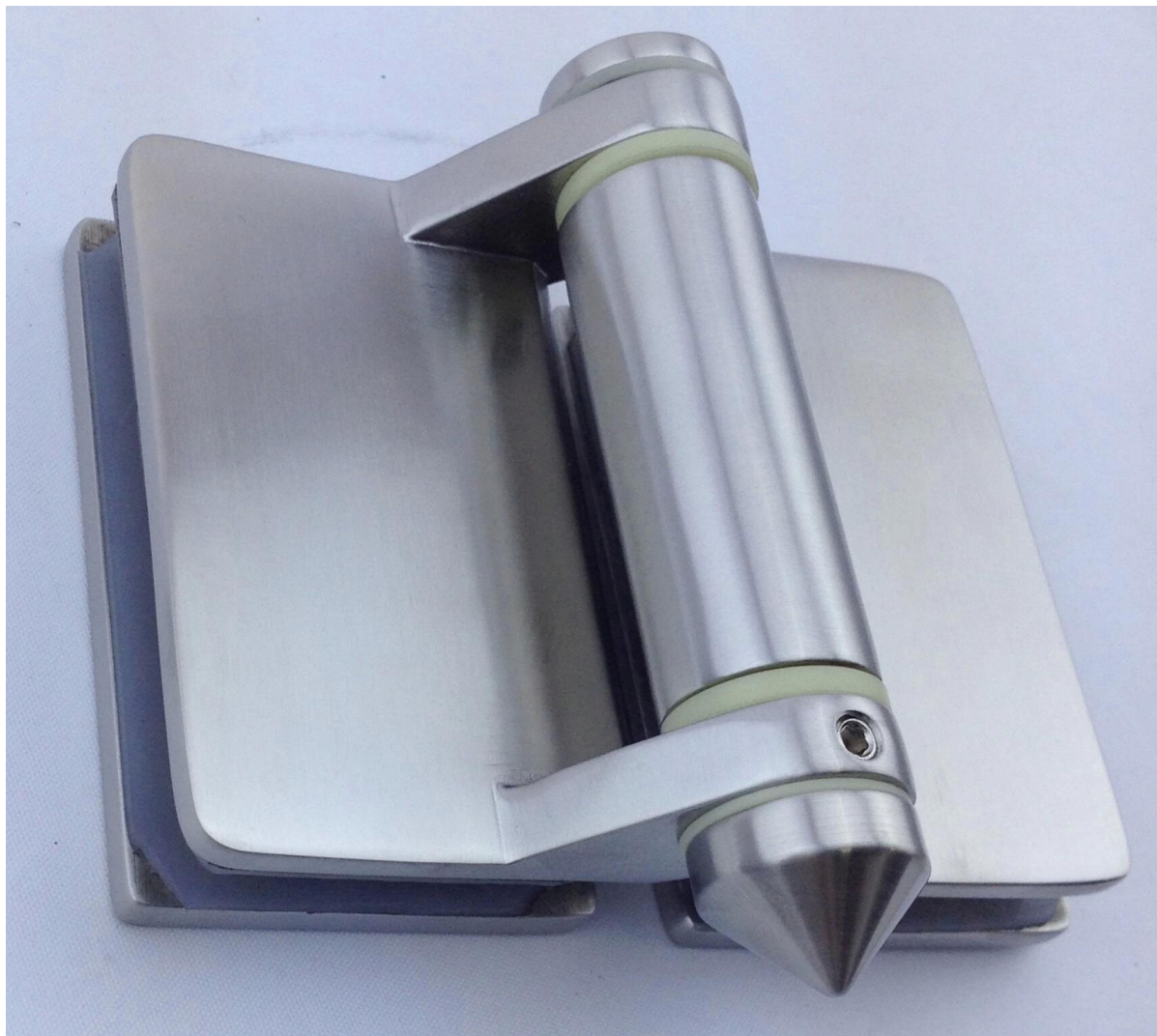
Стекло с круглой шарнирной петлей (диаметр круглой стойки 50,8 мм)
