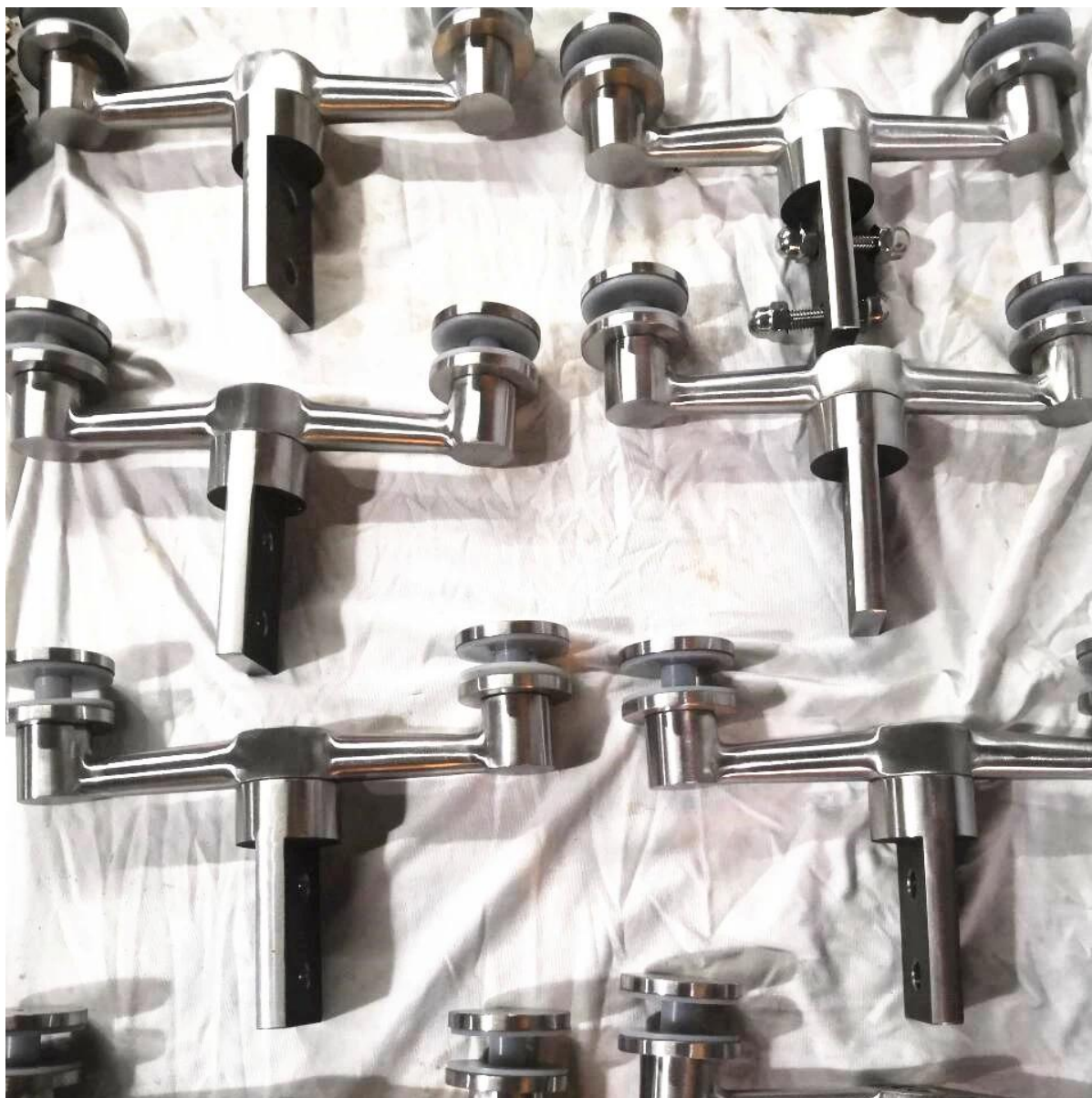
Фотография проекта стеклянного спайдерного фитинга для навесных стен -
