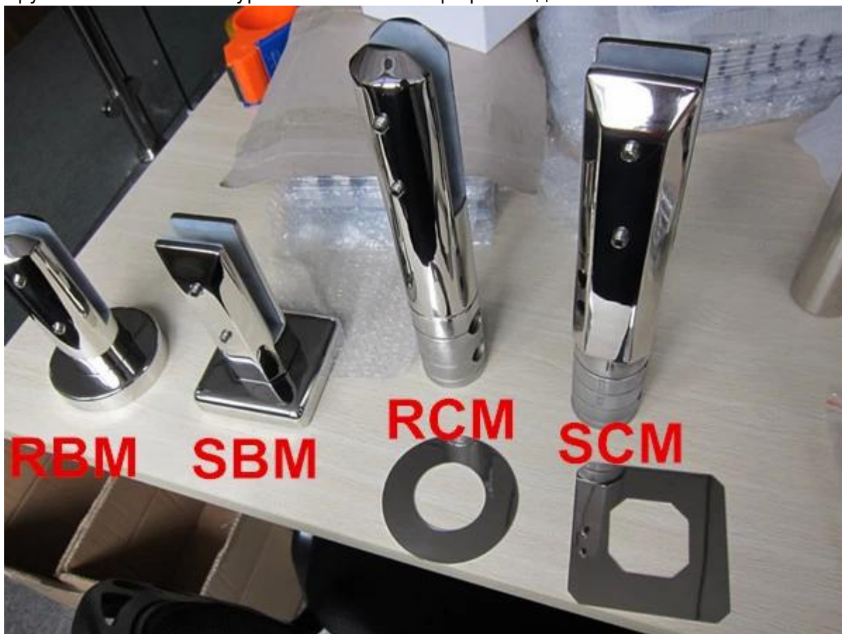
Круглый колонкового бурения бассейн забор кран модель. RCM
